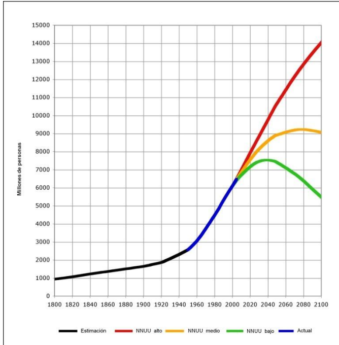
Previsions d'evolució de la població humana al món segons les Nacions Unides. Font: Population Division on the Department of Economic and Social Affairs of the United Nations Secretariat (2009). 'World Population Prospects: The 2008 Revision. Highlights'. New York: United Nations
